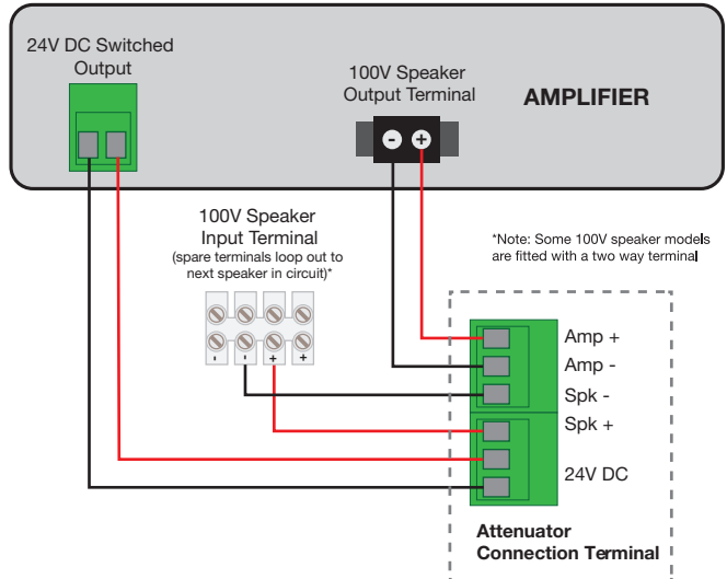
Wiring Diagram:
